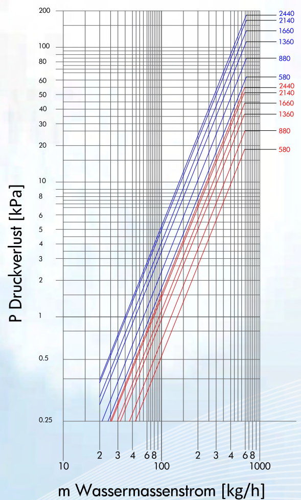
Wasserwiderstände 4-Leiter System
