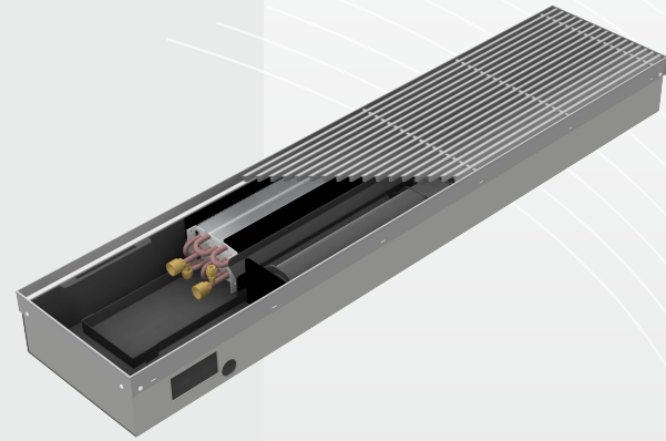
COLD-Modell betrieben mit Pumpenwarmwasser (PWW) und/oder Pumpenkaltwasser (PKW)
