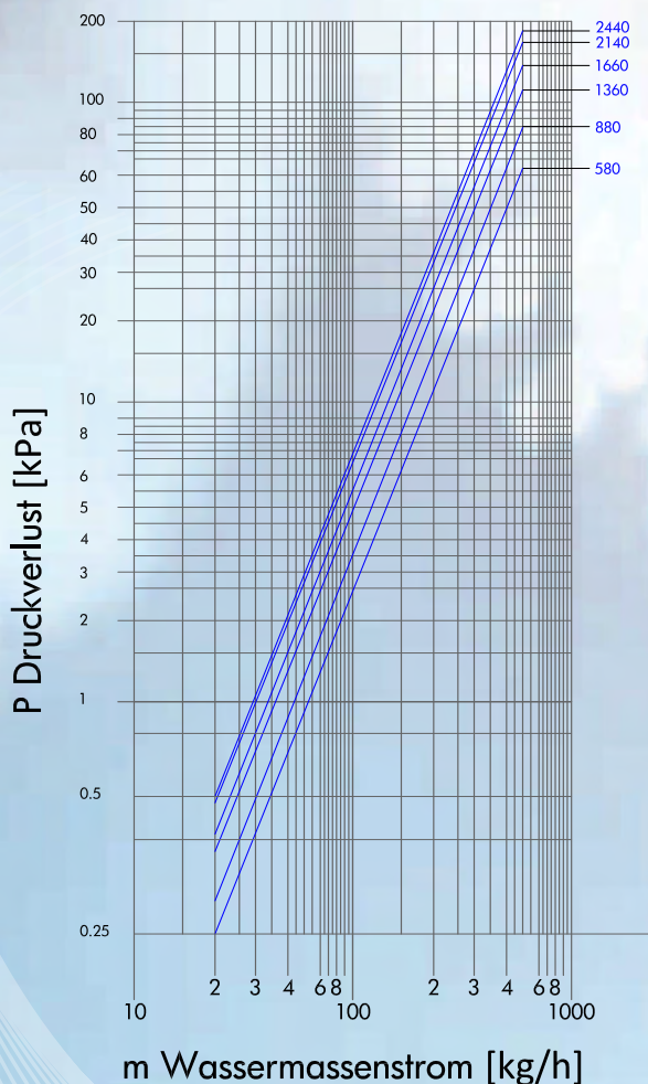
Wasserwiderstände 2-Leiter System
