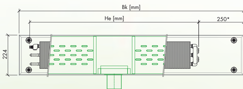
Grundriss auf Druckverteillblech. Anschluss seitlich
