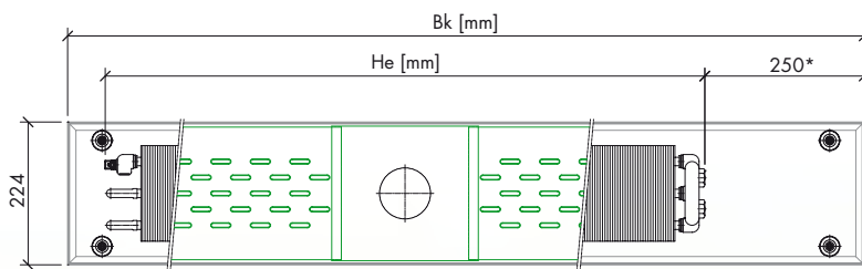
Grundriss auf Druckverteillblech. Anschluss von unten
