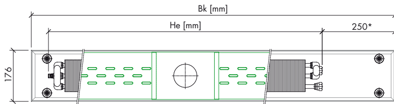
Grundriss auf Druckverteilech. Anschluss von unten
