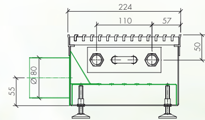
Anschlussmöglichkeit mit Stützen
