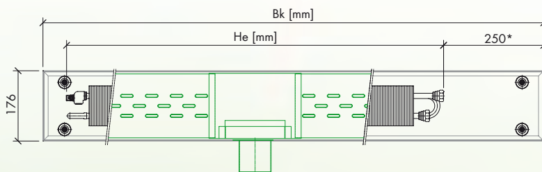
Grundriss auf Druckverteildblech. Anschluss seitlich
