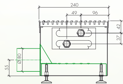
Anschlussmöglichkeit mit Stützen
