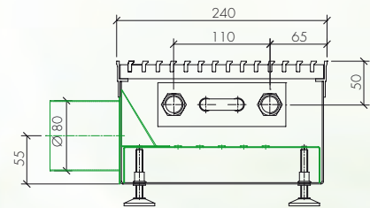
Anschlussmöglichkeit mit Stützen
