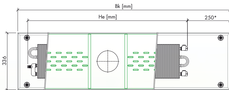
Grundriss auf Druckverteileblech. Anschluss von unten
