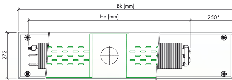
Grundriss auf Druckverteildblech. Anschluss von unten
