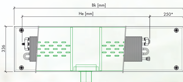
Grundriss auf Druckverteileblech. Anschluss seitlich
