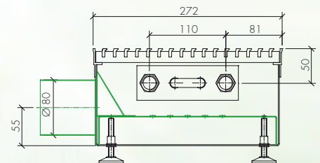
Anschlussmöglichkeit mit Stützen
