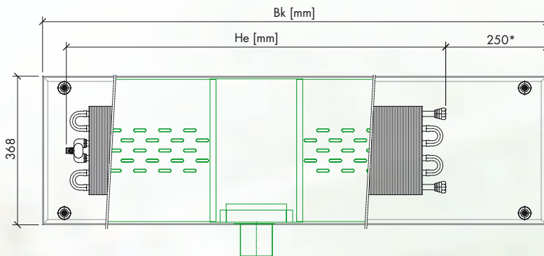
Grundriss auf Druckverteiltblech. Anschluss seitlich
