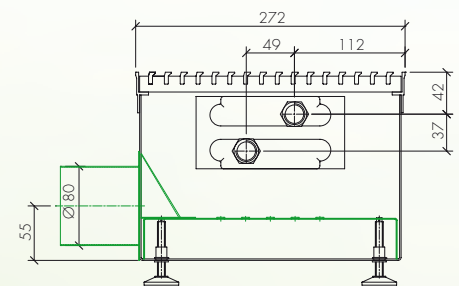
Anschlussmöglichkeit mit Stützen
