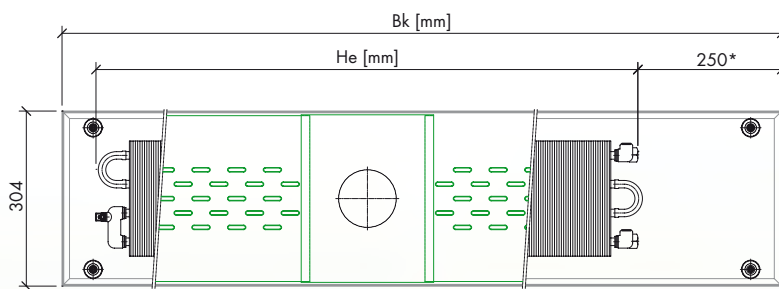
Grundriss auf Druckverteillblech. Anschluss von unten
