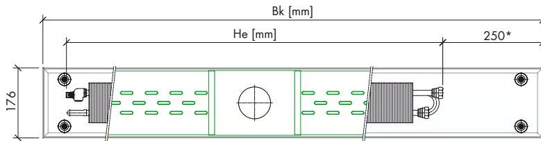
Grundriss auf Druckverteildblech. Anschluss von unten
