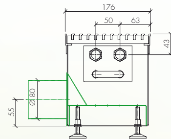
Anschlussmöglichkeit mit Stützen
