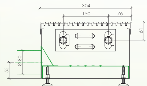
Anschlussmöglichkeit mit Stützen
