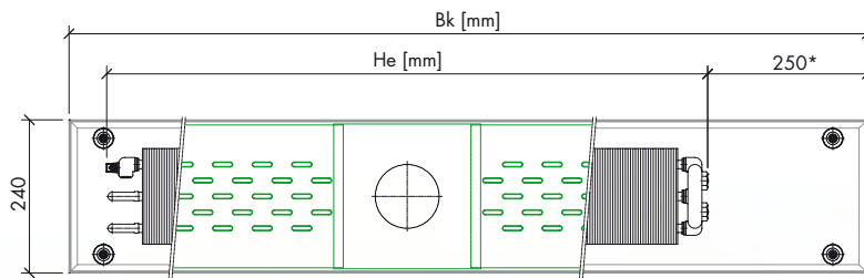
Grundriss auf Druckverteileblech. Anschluss von unten
