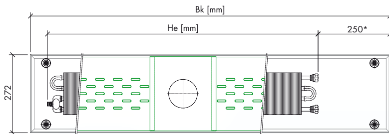
Grundriss auf Druckverteileblech. Anschluss von unten
