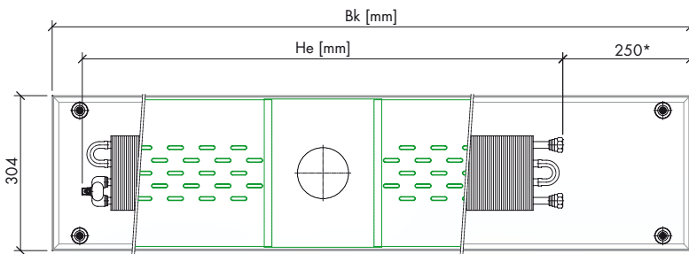
Grundriss auf Druckverteileblech. Anschluss von unten
