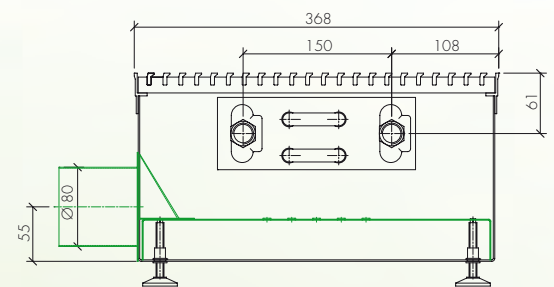
Anschlussmöglichkeit mit Stützen
