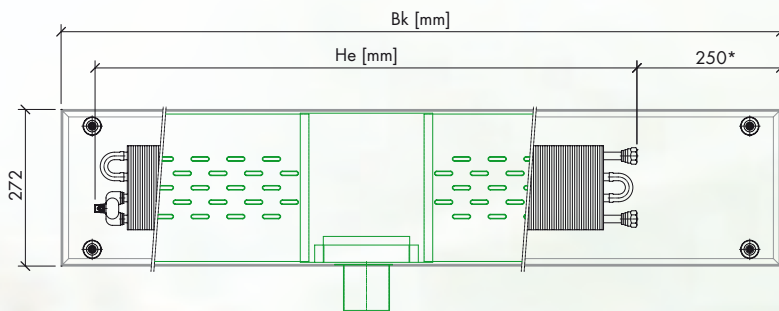
Grundriss auf Druckverteileblech. Anschluss seitlich
