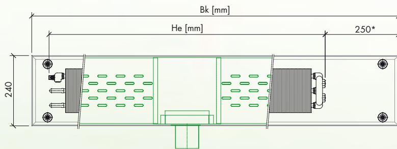
Grundriss auf Druckverteileblech. Anschluss seitlich
