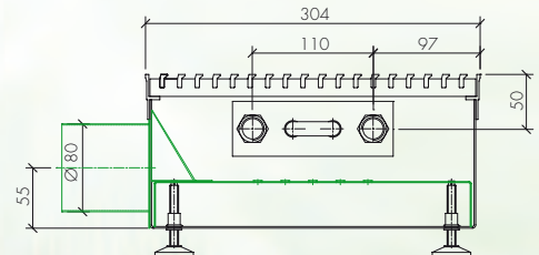
Anschlussmöglichkeit mit Stützen
