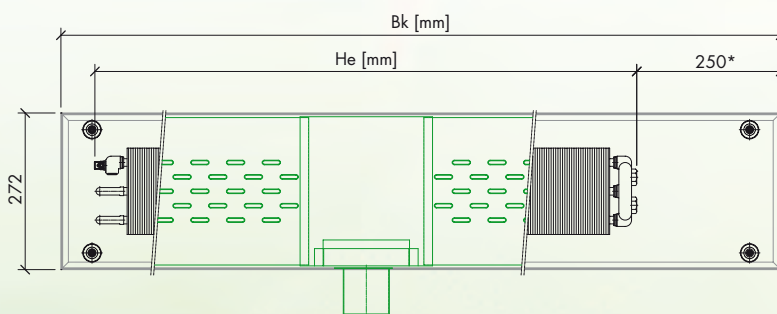
Grundriss auf Druckverteildblech. Anschluss seitlich
