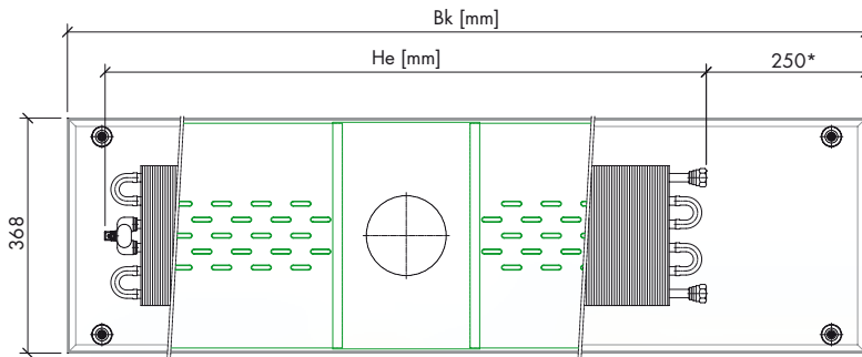
Grundriss auf Druckverteiltblech. Anschluss von unten
