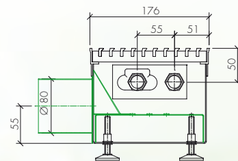
Anschlussmöglichkeit mit Stützen
