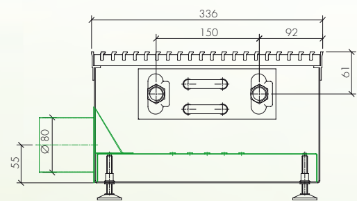
Anschlussmöglichkeit mit Stützen
