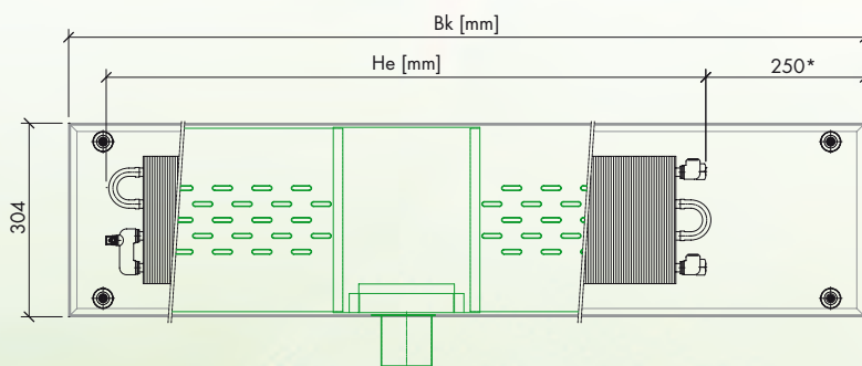
Grundriss auf Druckverteillblech. Anschluss seitlich
