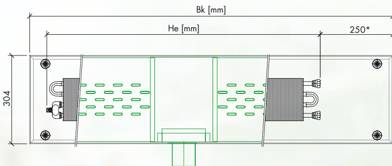
Grundriss auf Druckverteileblech. Anschluss seitlich
