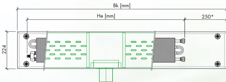
Grundriss auf Druckverteillech. Anschluss seitlich
