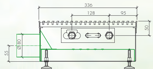
Anschlussmöglichkeit mit Stützen
