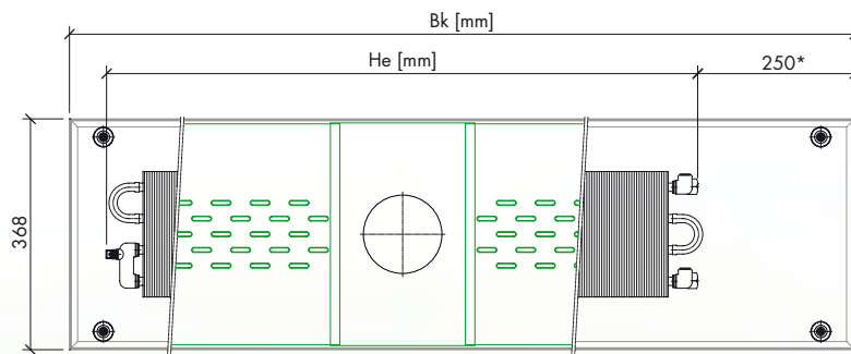
Grundriss auf Druckverteildblech. Anschluss von unten
