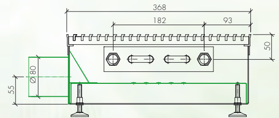
Anschlussmöglichkeit mit Stützen
