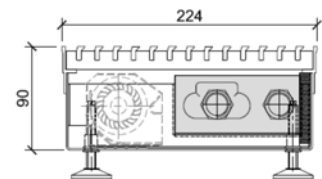
Modell FAN 224-090 (Anschluss seitlich)
