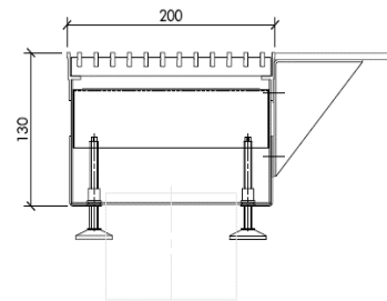
Modell SOL FRE200 - 130 (Anschluss von unten)
