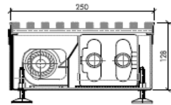
Modell COLD 250-128-T2
