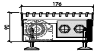
Modell FAN 176-090 (Anschluss seitlich)
