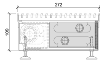
Modell FAN 272-109 (Anschluss seitlich)
