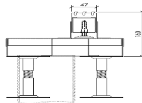
Modell SOL 47 - 160 (Anschluss von unten)
