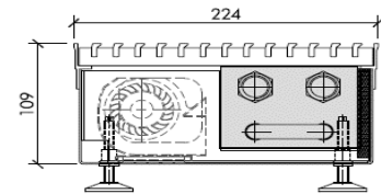
Modell FAN 224 – 109 (Anschluss seitlich)
