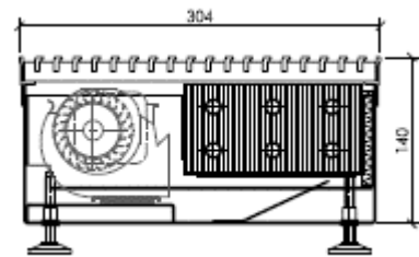
Modell FAN 304-140 (Anschluss seitlich)
