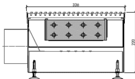
Modèle ARIA 336-220
