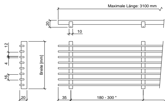
Grilles linéaires 1610 -B
