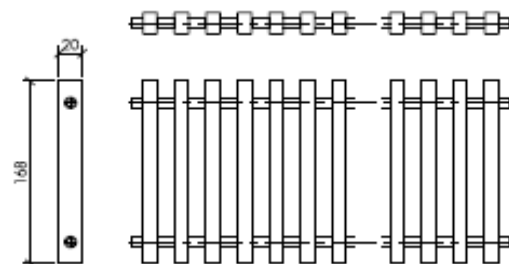
Grille enroulable Legna Latus 1227-B
