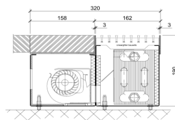
Modèle FAN 320-190
